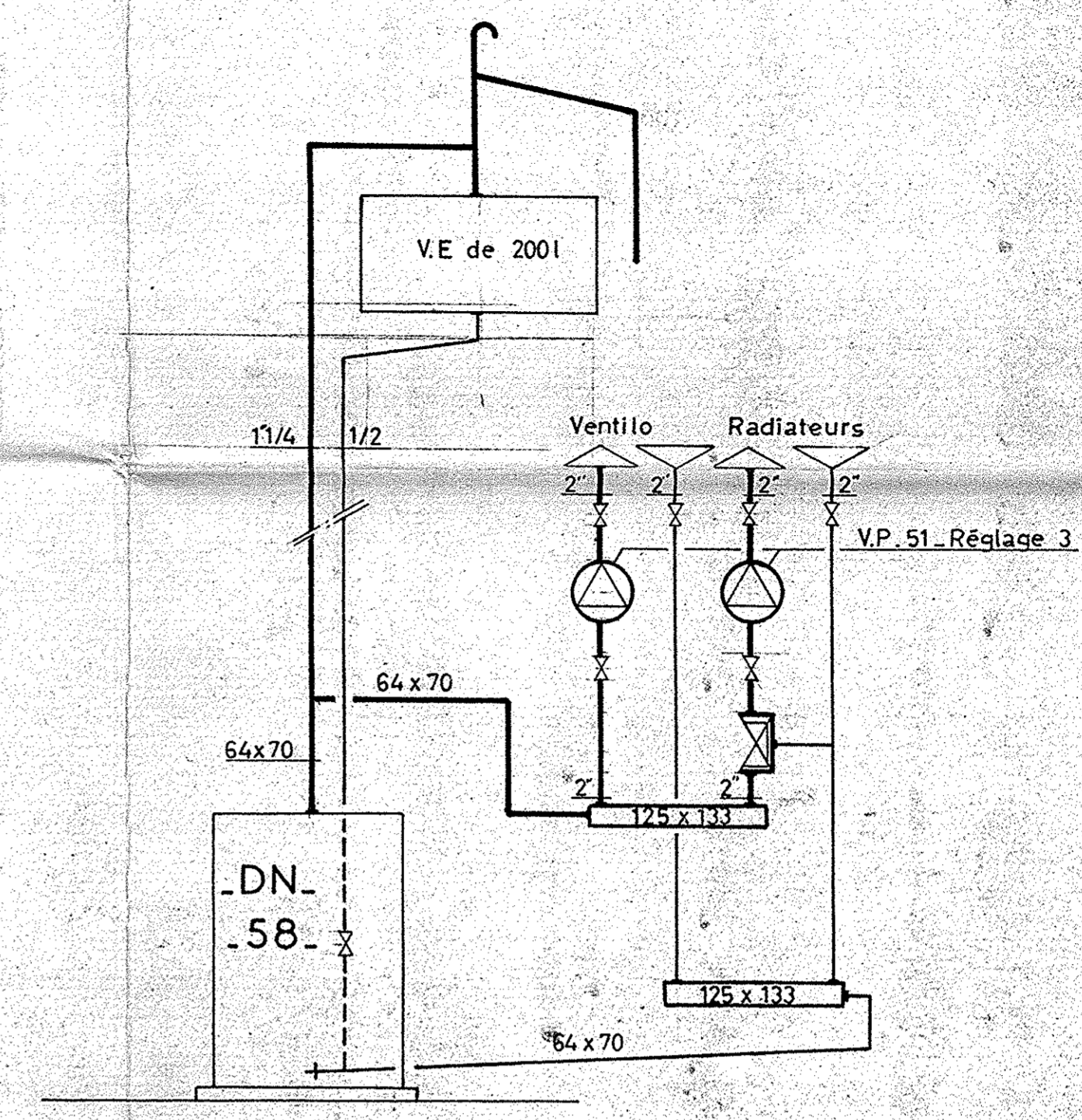
SCHEMA DE CHAUFFERIE
